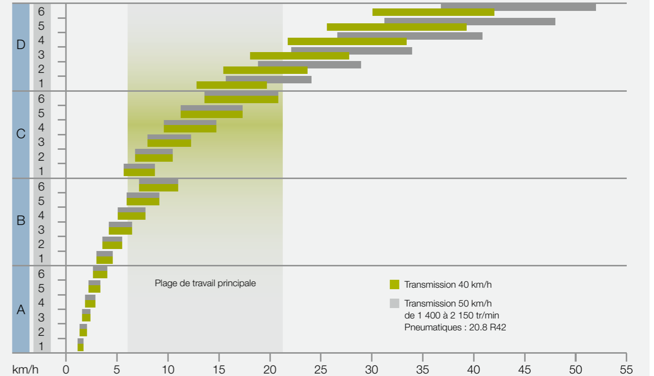
HEXASHIFT : 24 rapports pour un étagement optimal de la transmission
